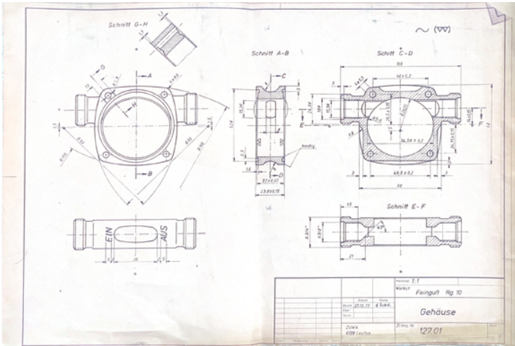
1977 Technische Zeichnung angefertigt mit Bleistift und Tusche
