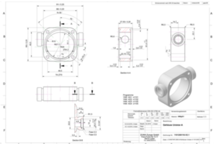
2016 Technische Zeichnung angefertigt mit CAD mit 3D-Modell
